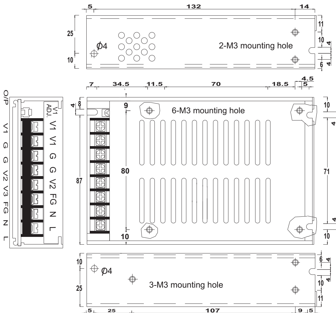
機構圖
